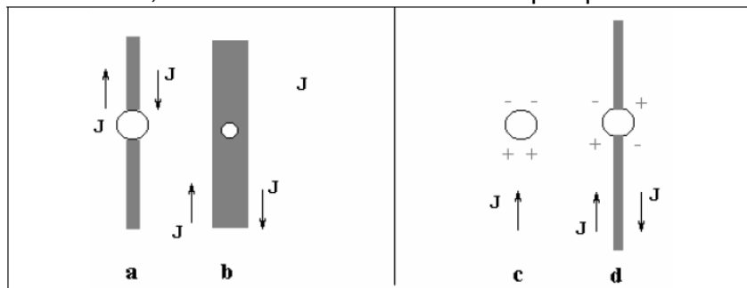
Figura 1. As figuras (a) e (b) mostram que a energia total da parede é reduzida. Em (c) e (d) é mostrado a reconfiguração do polos magnéticos quando a parede ancora numa inclusão. A energia Magnetostática é menor na situação (d) do que em (c).
