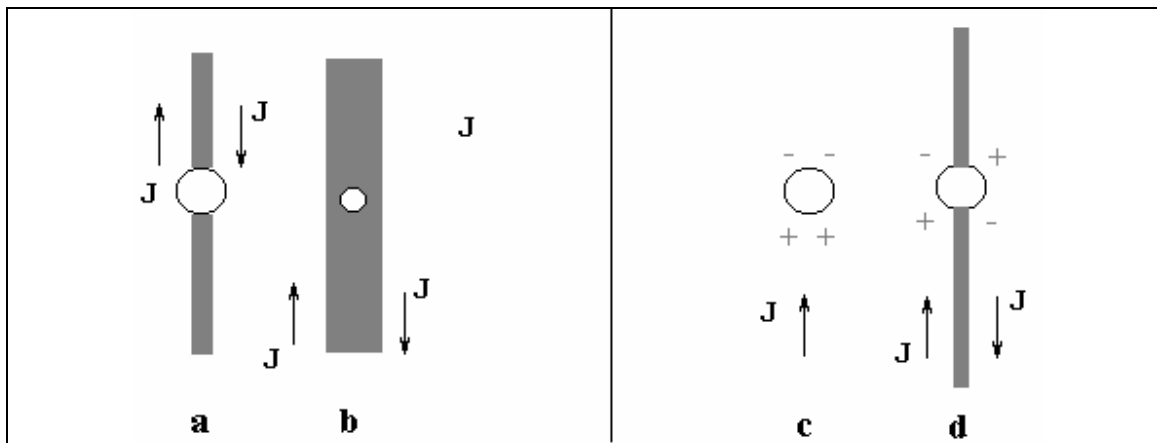
Fig.1) – As figuras (a) e (b) mostram que a energia total da parede é reduzida. Em (c) e (d) é mostrado a reconfiguração do polos magnéticos quando a parede ancora numa inclusão. A energia Magnetostática é menor na situação (d) do que em (c).
